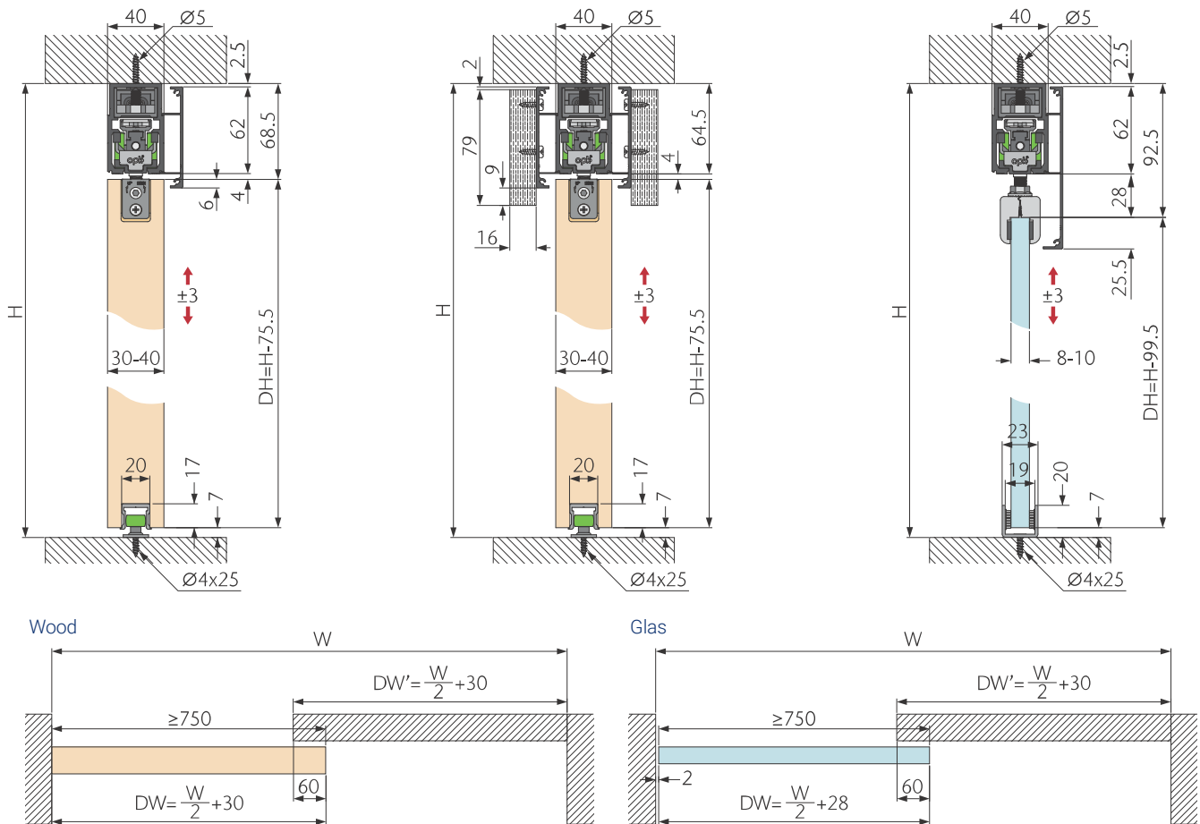
Technische Zeichnung / Technical Drawing
