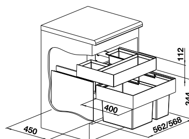
Beispiel Maßskizze 3377518725
