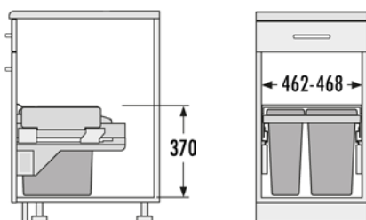
Maßzeichnung 3387100796
