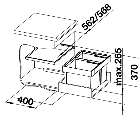
Ansicht und Einbausituation Modell 3377521471
