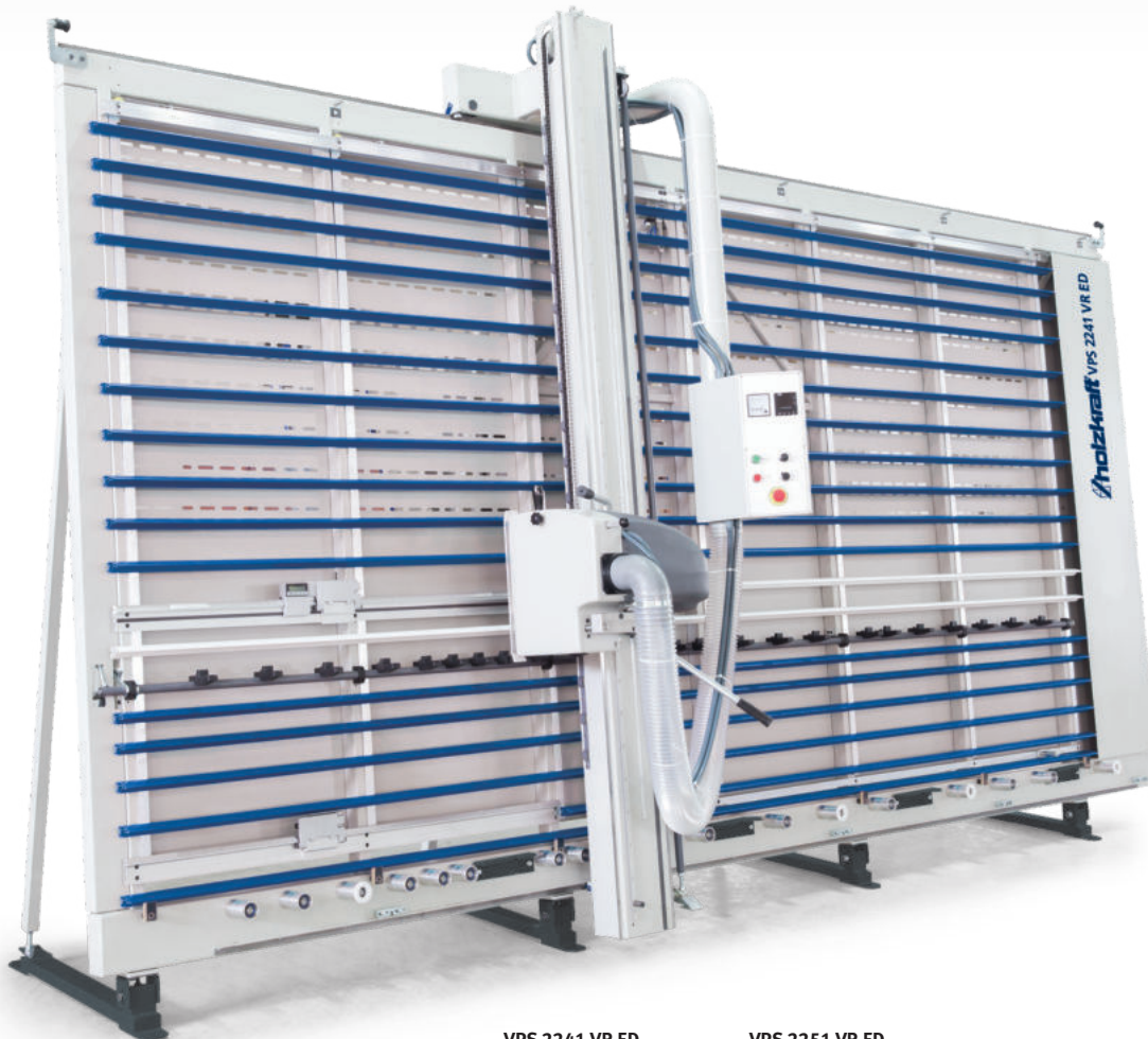
▶ Vertikalschnitt
