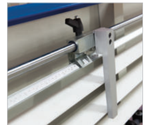
▶ Lineal zur Längeneinstellung beim Vertikalschnitt
