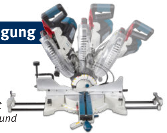
Ausziehbare Anlageschienen und ausziehbarer Tisch
